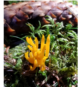
Clavaire
